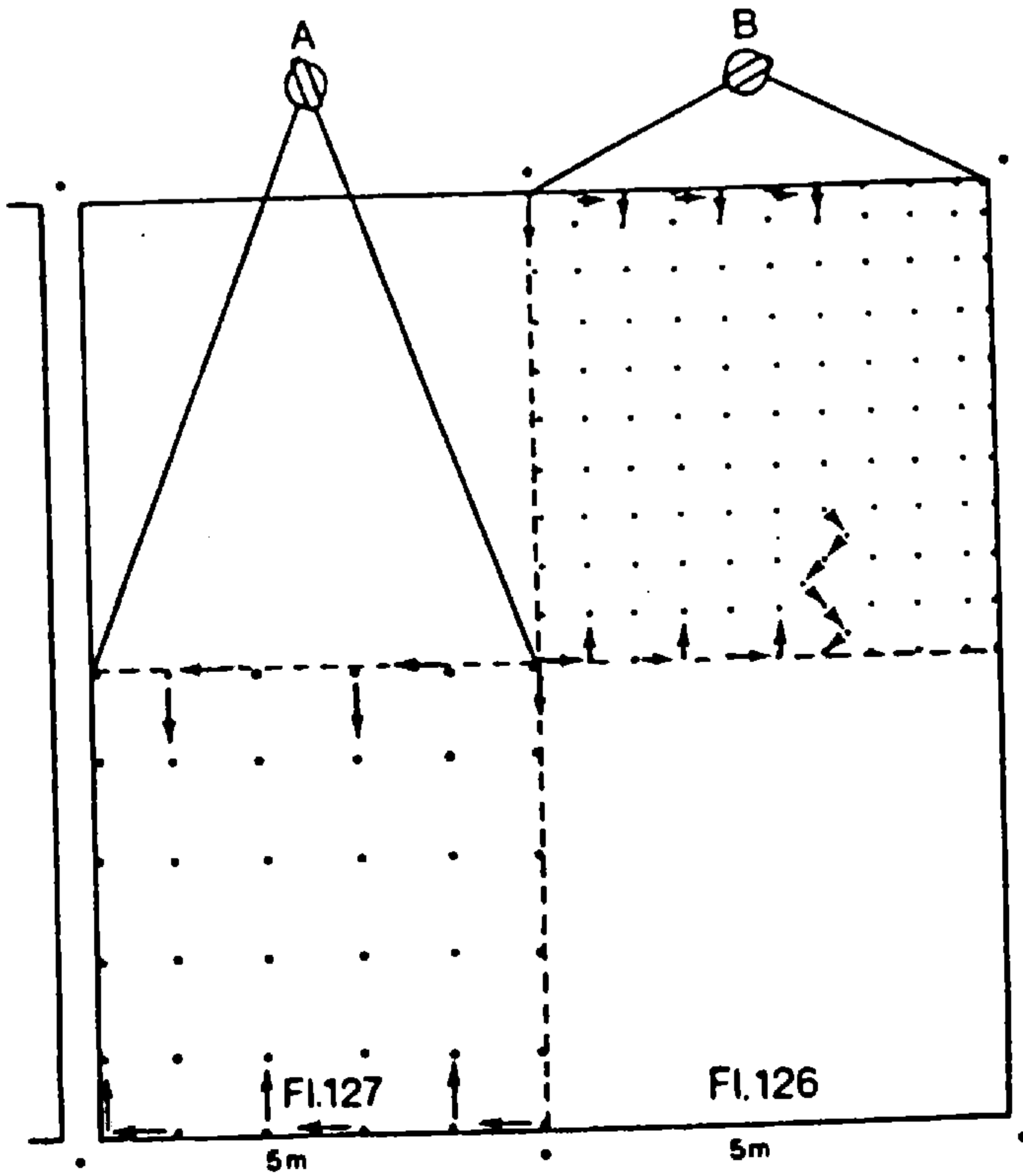
(شكل ٧) طريقة قياس تسوية الأرض
